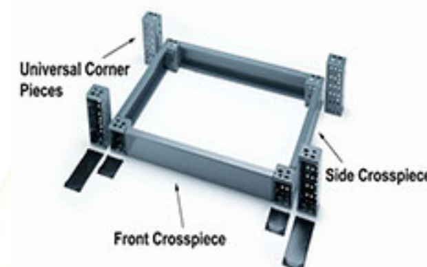
組合式腳座 - 普通鋼；顏色深灰色 Modular Plinth - Sheet Steel ; Colour RAL7025
