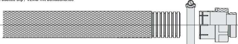
VEMD with Jubilee clip / VEMD mit Schlauchbride
